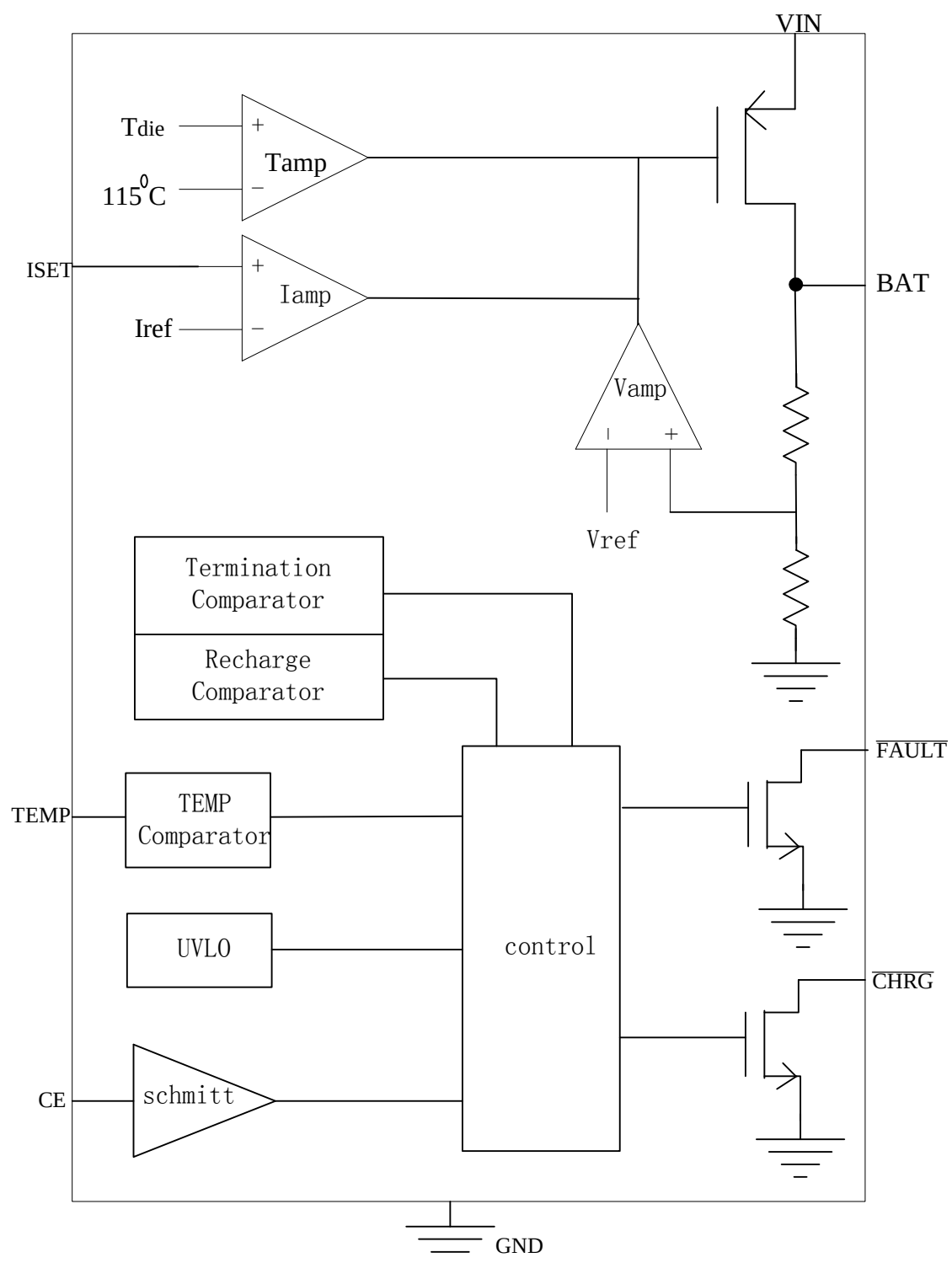
图 2 功能框图
