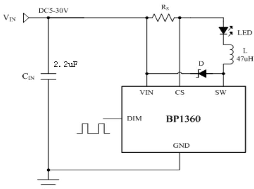
图表 1 典型应用图
